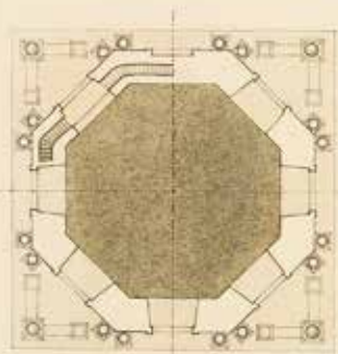
ПЛАН ВОСЬМЕРНИКА
