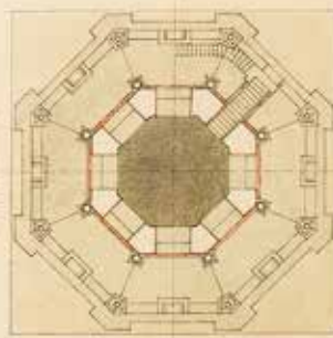
ПЛАН КОЛОКОЛЬНИ
